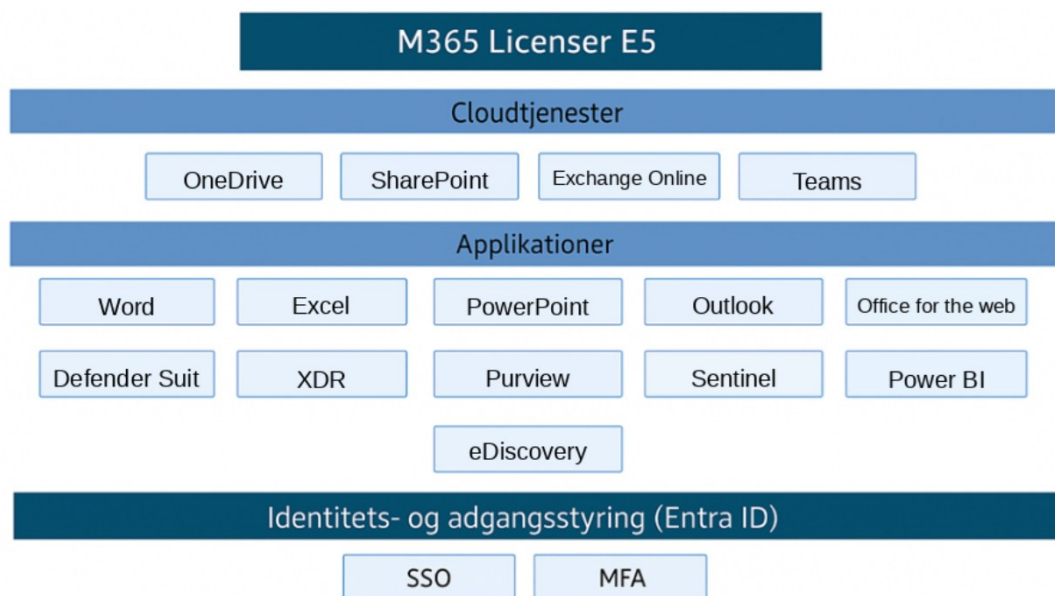
Figur 1 M365-værktøjer
